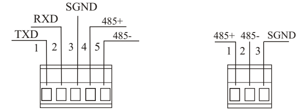
Fig 3. RS-232C/RS-485 input interface Fig 4. RS-485 output interface
